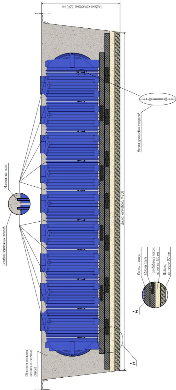
Схема монтажа РТ45
