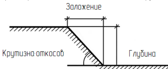
Рисунок 2. Крутизна откосов котлована
