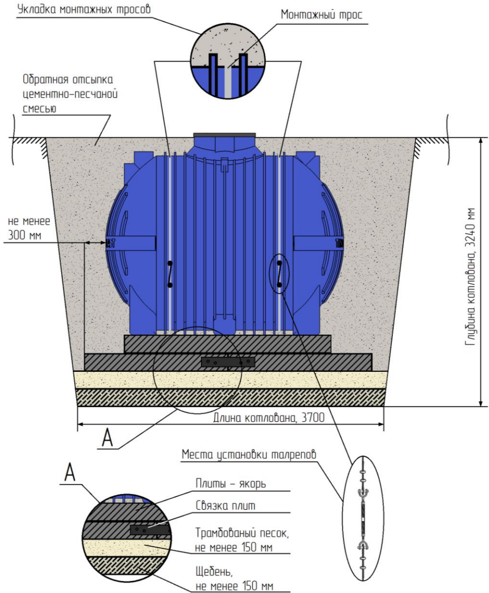
Схема монтажа РТ10
